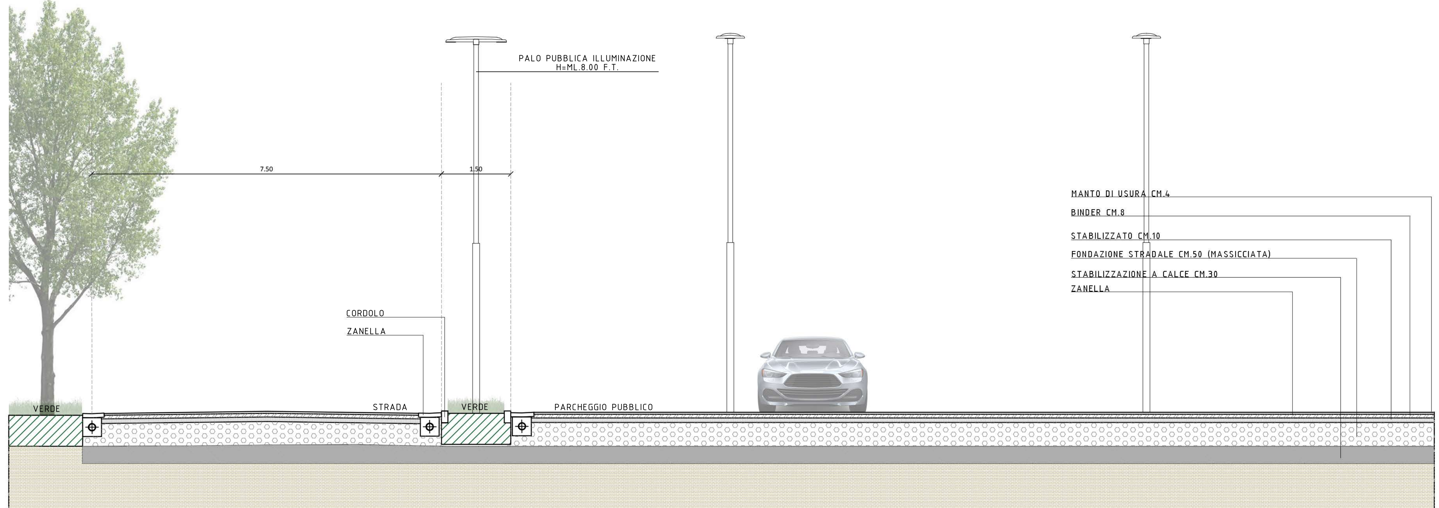
SEZIONE B-B _ 1:50
