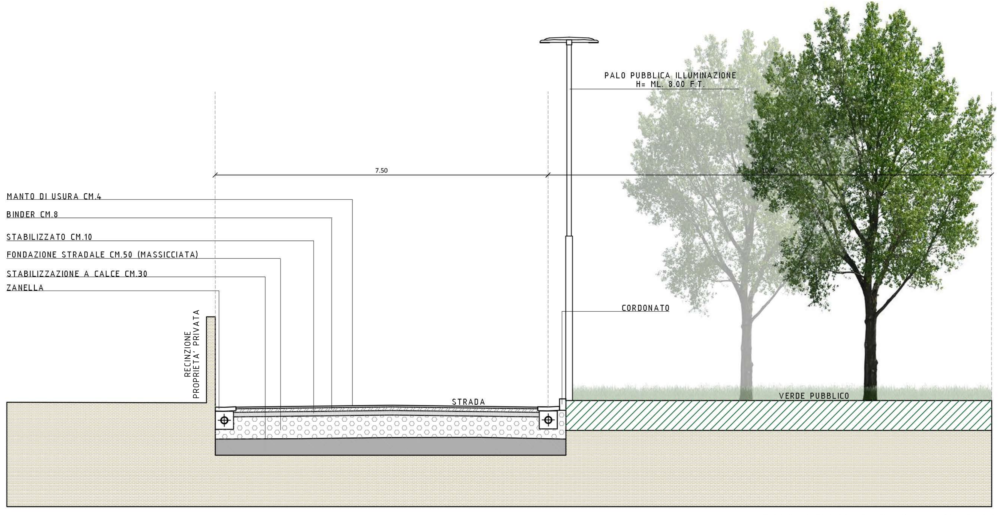
SEZIONE A-A _ 1:50
